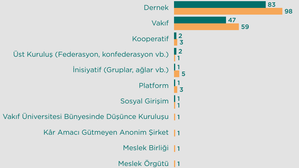
GRAFİK 1. STK'LARIN KURULUŞ TÜRÜ
